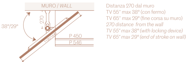
ROTAZIONE SUPPORTO TV / TV SUPPORT ROTATION
