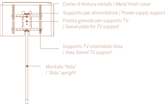
ROTAZIONE SUPPORTO TV / TV SUPPORT ROTATION
